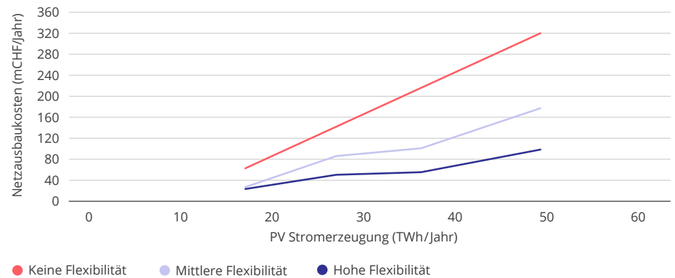
Abbildung 8: Zusätzliche Netzausbaukosten in Abhängigkeit der PV-Stromerzeugung und verfügbarer Flexibilität. Modernisierung des bestehenden Netzes ist hier nicht berücksichtigt.
